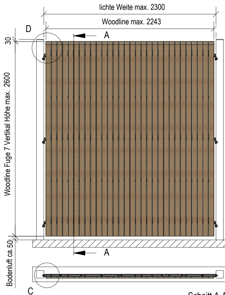
Schnitt A-A
