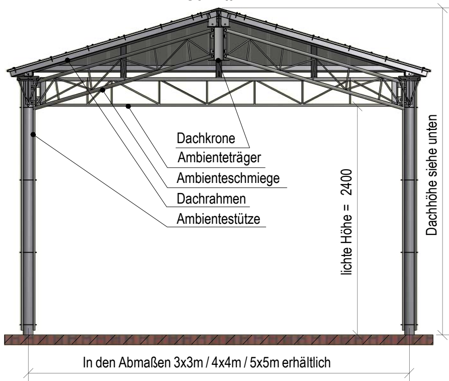
Schnitt A-A
