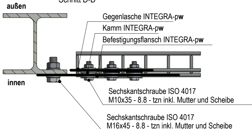
Schnitt D-D
