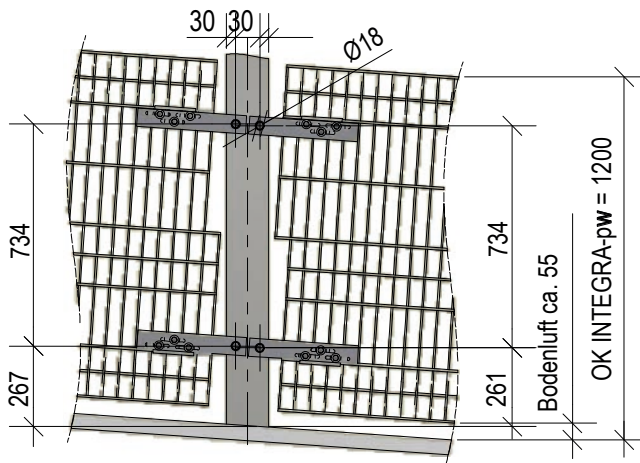
Bohrbild für Rampenmatte - Gefälle 10 % - 16 %
