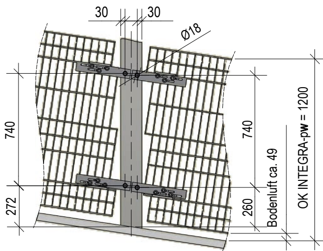
Bohrbild für Rampenmatte - Gefälle 10 % - 16 %
