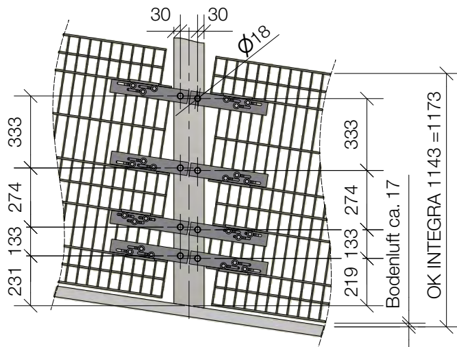
Bohrbild für Rampenmatte - Gefälle 10 % - 16 %
