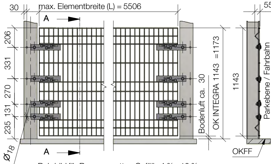
Bohrbild für Rampenmatte - Gefälle 4 % - 10 %
