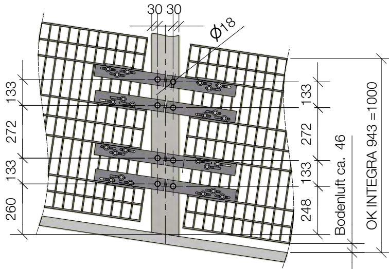
Bohrbild für Rampenmatte - Gefälle 10 % - 16 %
