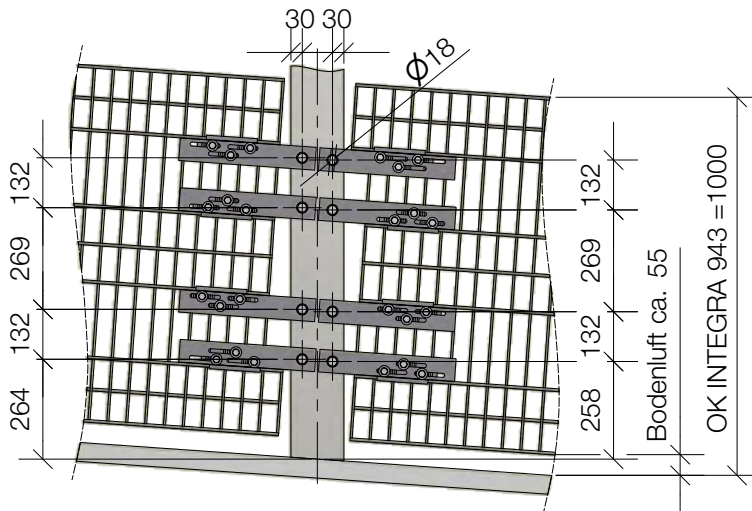
Bohrbild für Rampenmatte - Gefälle 10 % - 16 %
