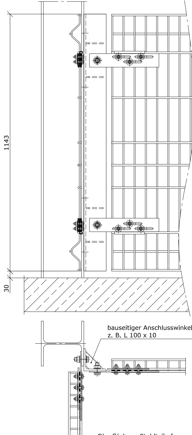
Anschlussdetail Stützenverdrehung (schraubbar) bauseitige und statisch ausreichend dimensionierte Anschlusswinkel
